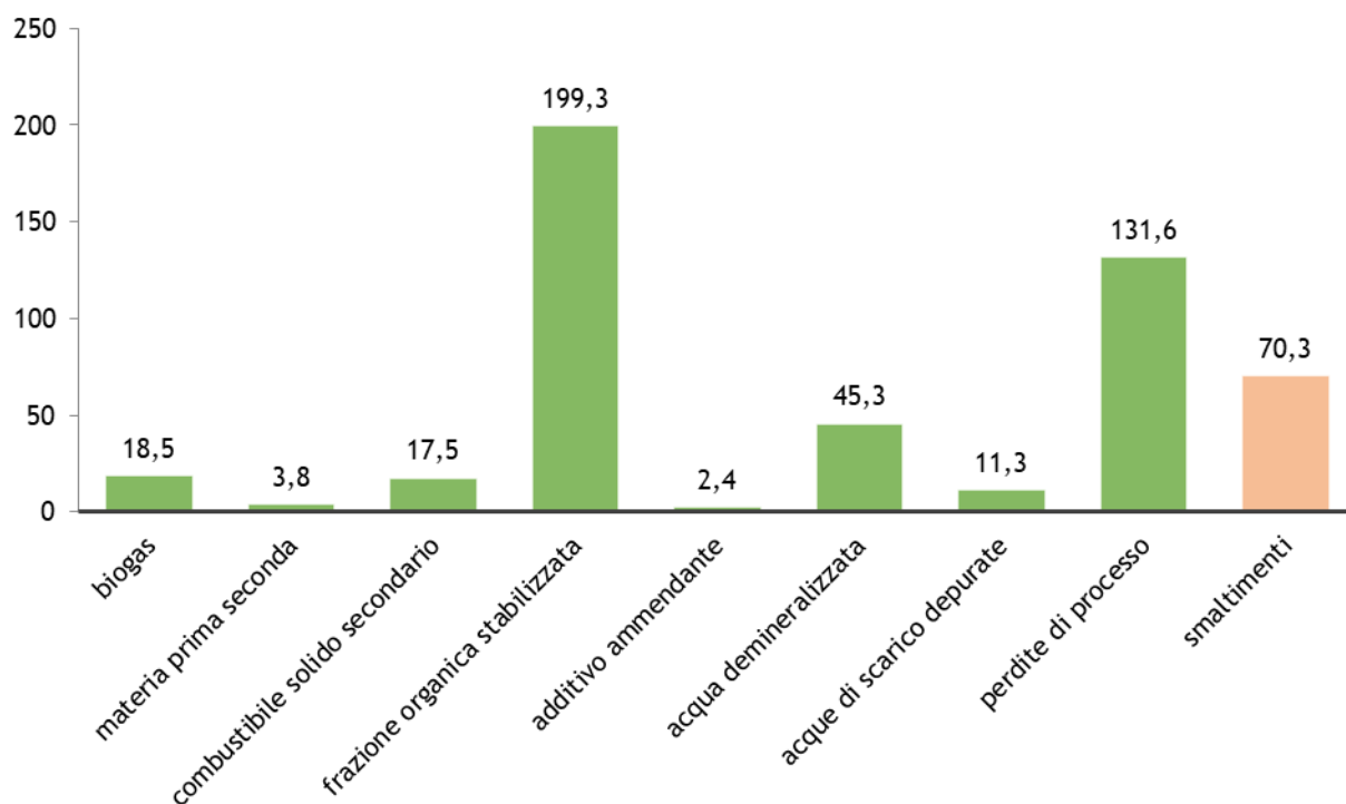
Figura I31 – Flussi in uscita a regime Scenario 2 - Target (t/000)
