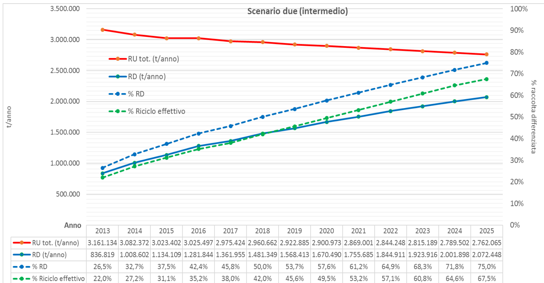
Figura 16– Flussi di RU attesi con lo SCENARIO DUE (INTERMEDIO) nel Lazio al 2025
