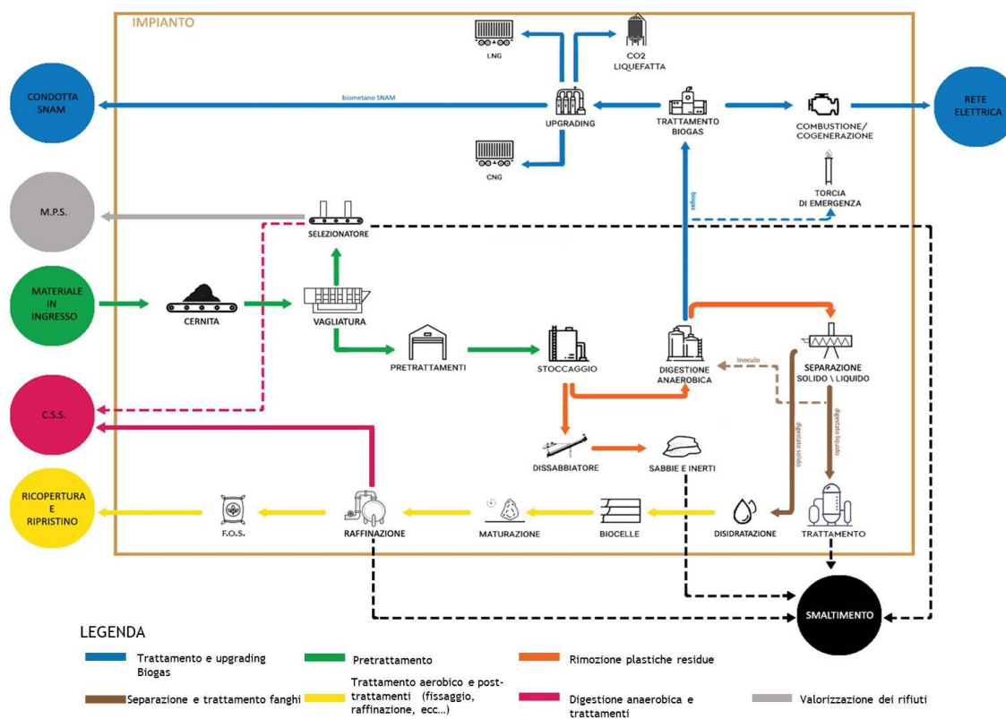
Figura 129 – Layout di impianto
