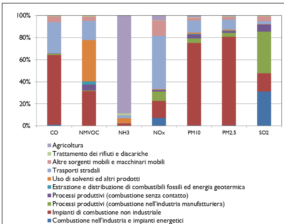
Figura 43 - Emissioni per macrosettore – LAZIO 2015 (t)
