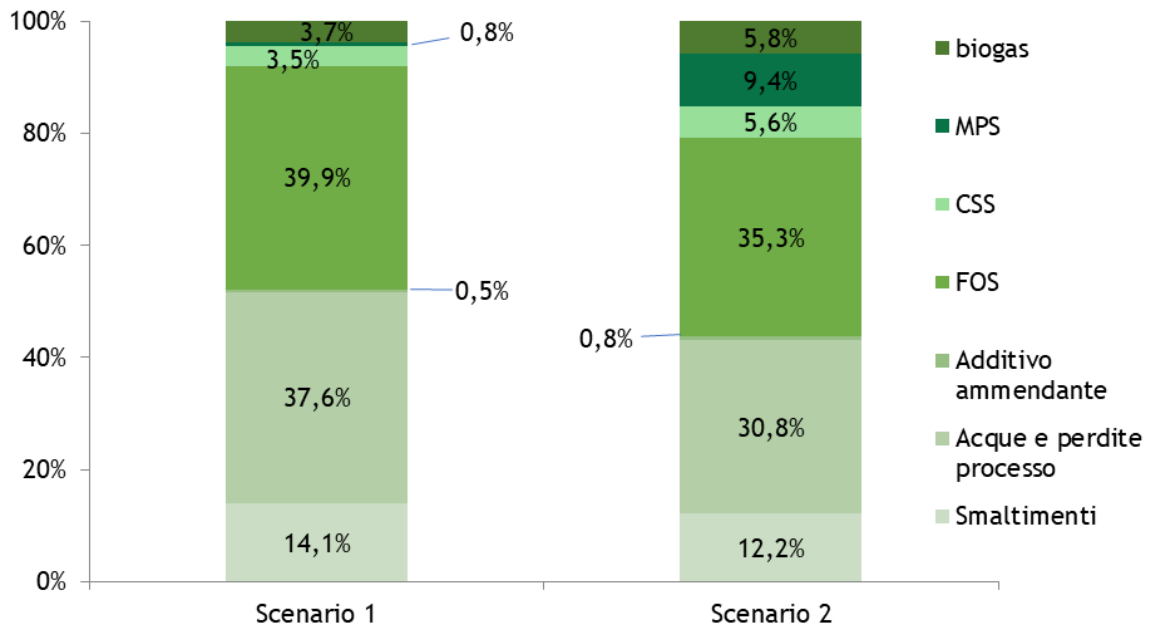
Figura 132 – Confronto tra i flussi in uscita nei due scenari
