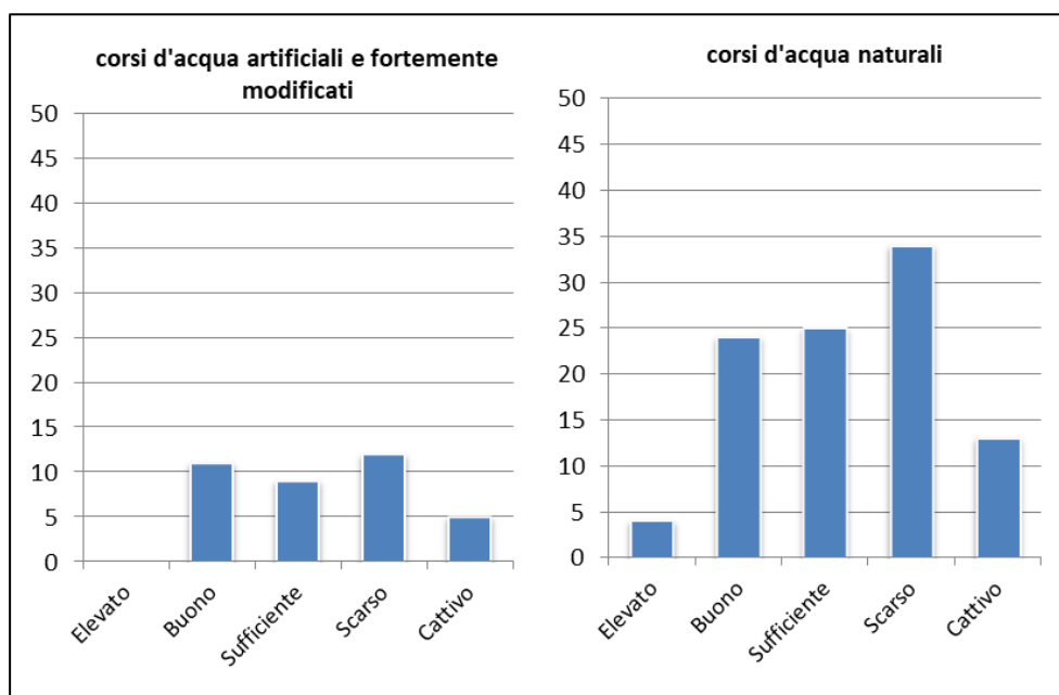
Figura 46– Stato Ecologico dei corsi d'acqua
