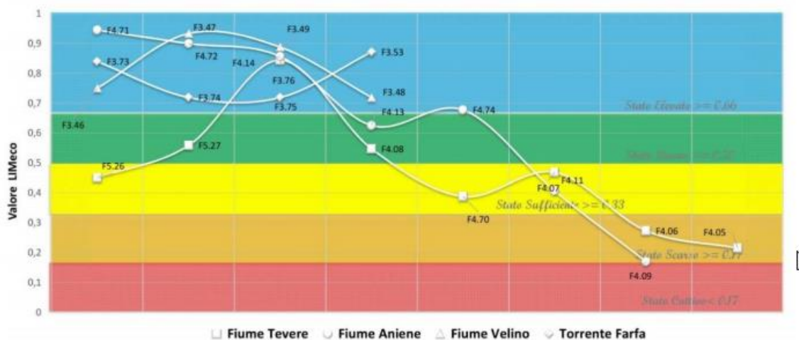
Figura 45– Distribuzione dell'indice trofico LIMeco sulle aste dei fiumi principali del bacino del Tevere (2015 -2017)
