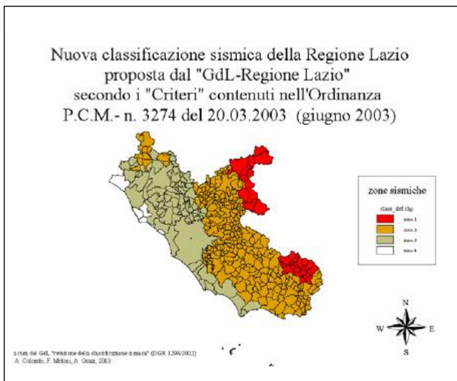
Figura 48– Classificazione sismica della Regione Lazio
