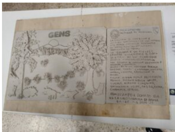
mappa tridimensionale della Caldara di Manziana
